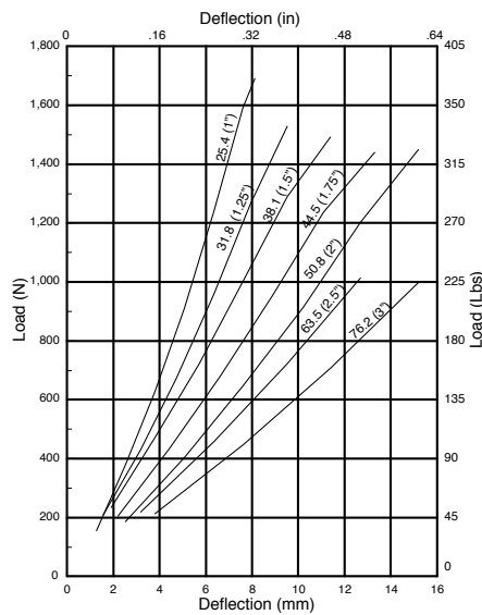
FIG. 8 P0875-XXXX-60A
